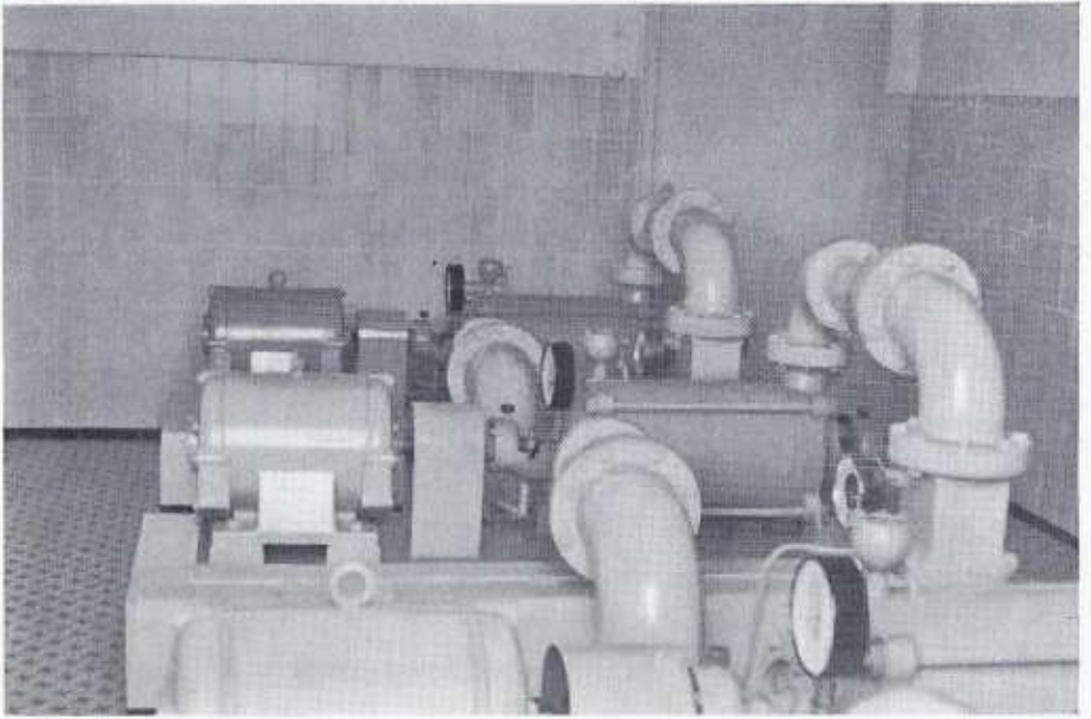
Hauptpumpanlage
