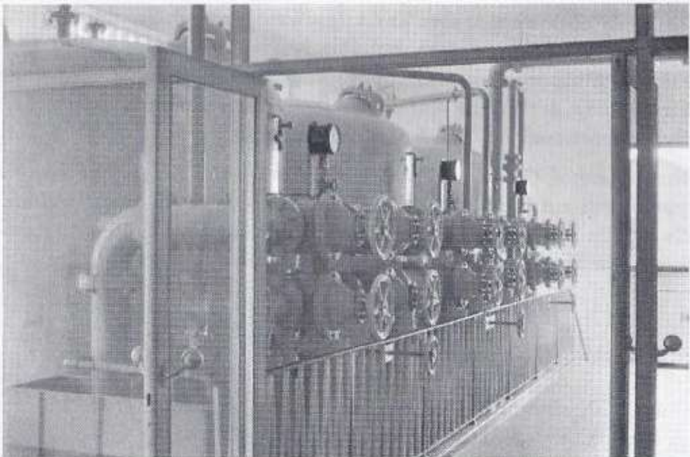
Teilansicht der Aufbereitungsanlage (Filterkesseln)
